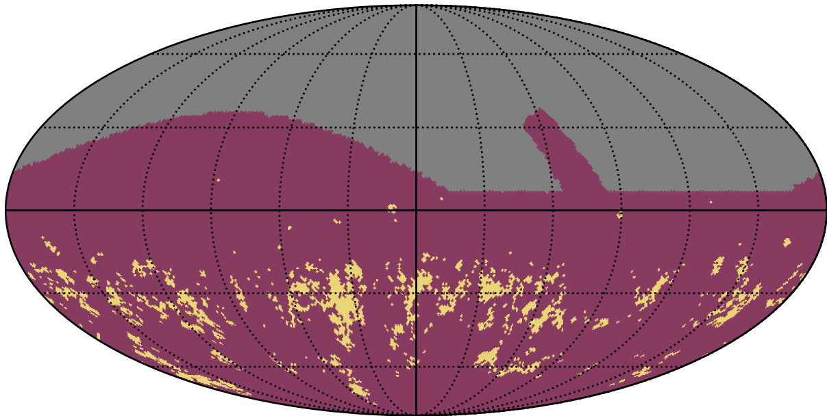
retro_baseline_v2.0_10yrs r band: Gaps_7hr
