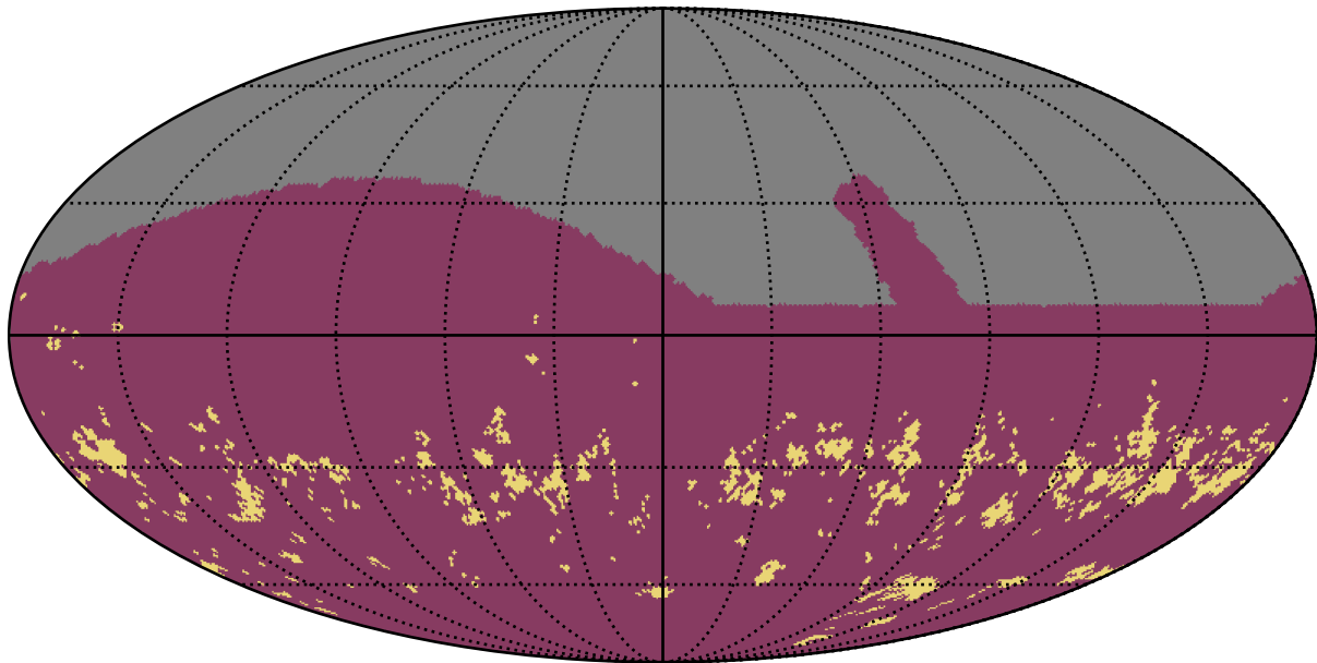
retro_baseline_v2.0_10yrs i band: Gaps_7hr
