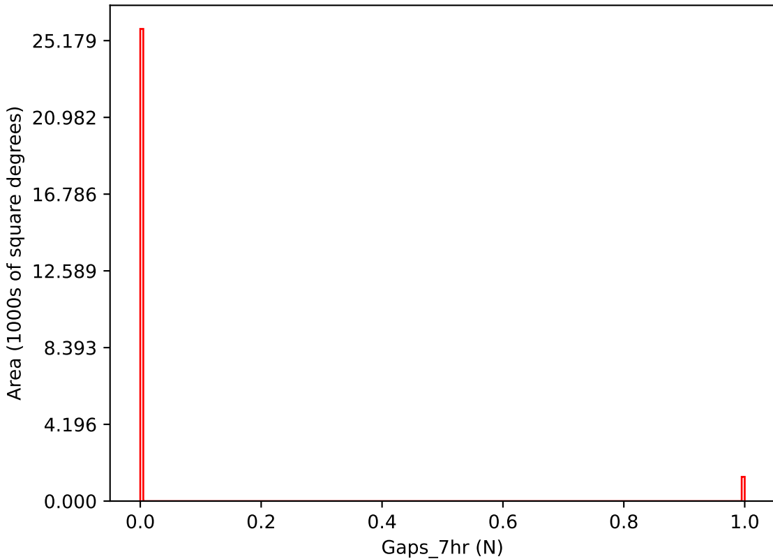
retro_baseline_v2.0_10yrs i band: Gaps_7hr
