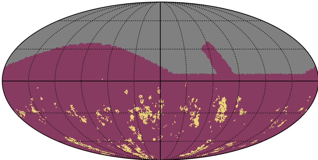
retro_baseline_v2.0_10yrs g band: Gaps_7hr
