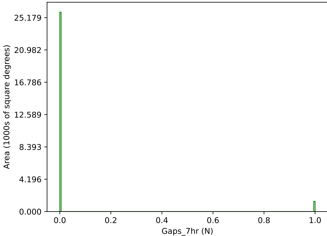
retro_baseline_v2.0_10yrs g band: Gaps_7hr
