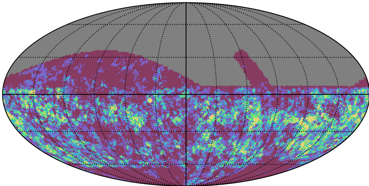
retro_baseline_v2.0_10yrs z band: Gaps_3hr
