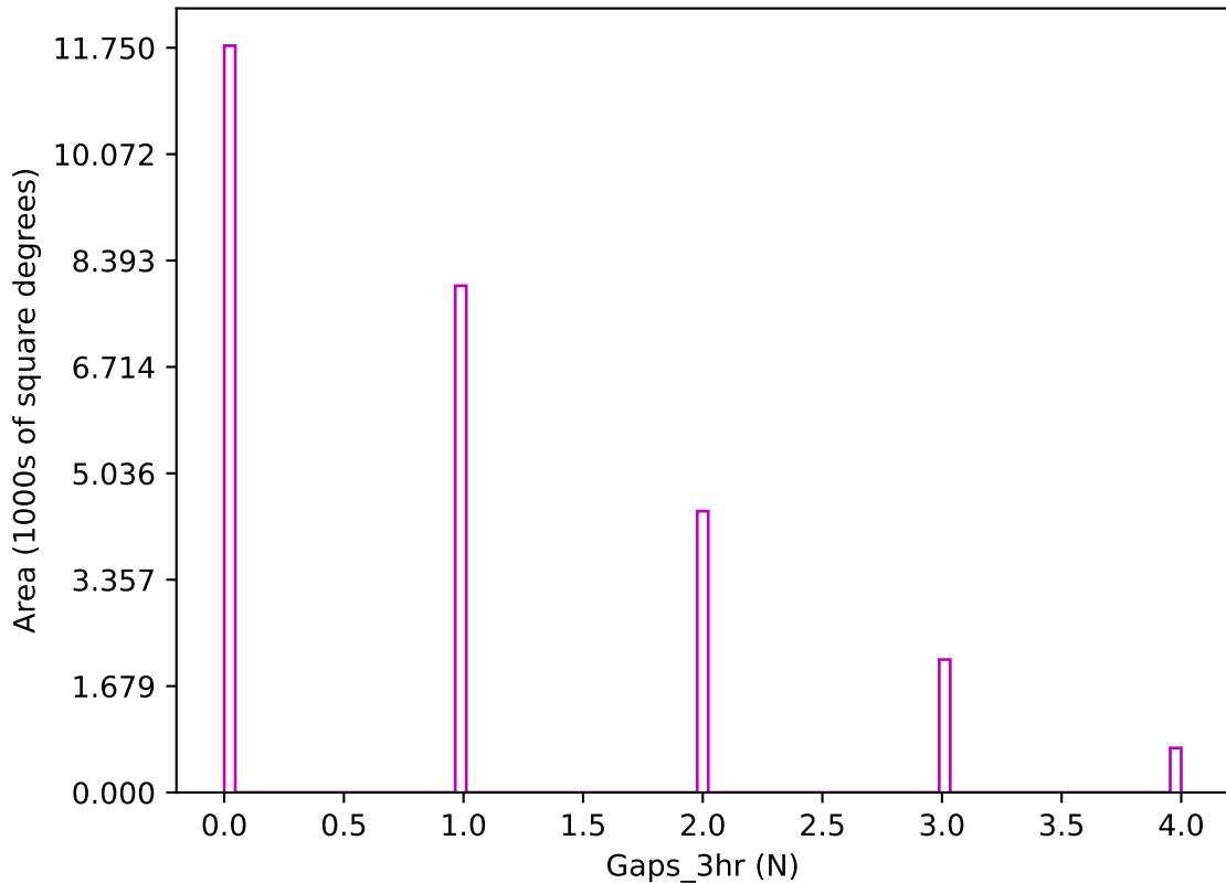
retro_baseline_v2.0_10yrs z band: Gaps_3hr
