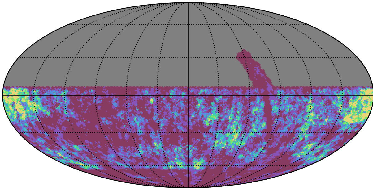
retro_baseline_v2.0_10yrs y band: Gaps_3hr
