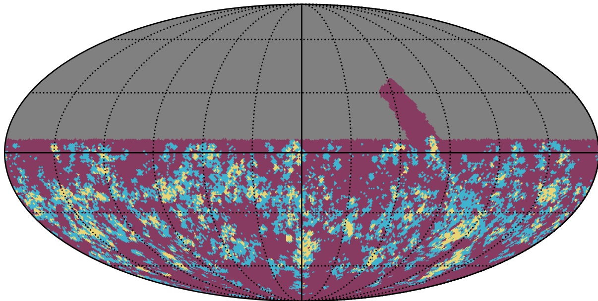
retro_baseline_v2.0_10yrs u band: Gaps_3hr
