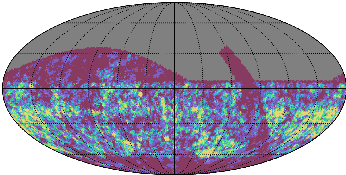
retro_baseline_v2.0_10yrs r band: Gaps_3hr
