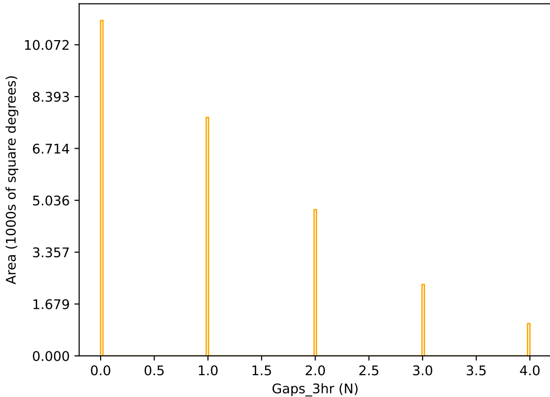
retro_baseline_v2.0_10yrs r band: Gaps_3hr
