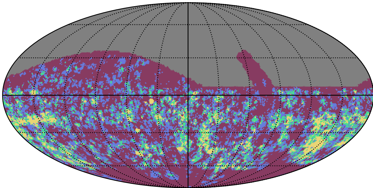
retro_baseline_v2.0_10yrs i band: Gaps_3hr
