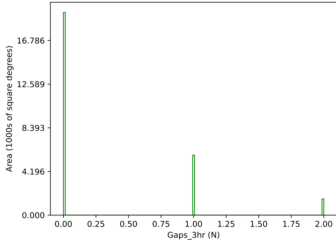
retro_baseline_v2.0_10yrs g band: Gaps_3hr
