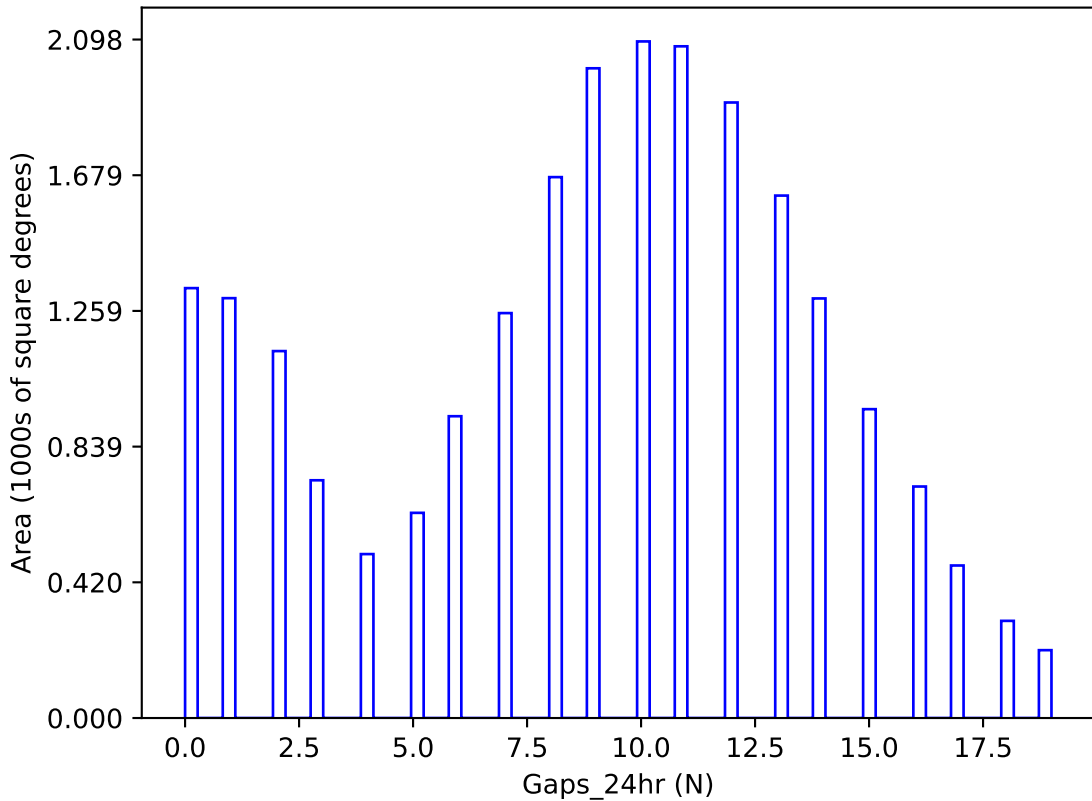
retro_baseline_v2.0_10yrs y band: Gaps_24hr
