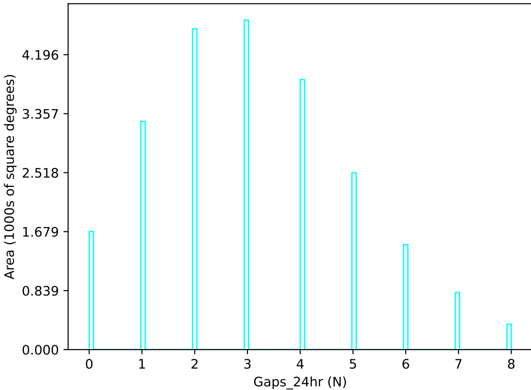
retro_baseline_v2.0_10yrs u band: Gaps_24hr
