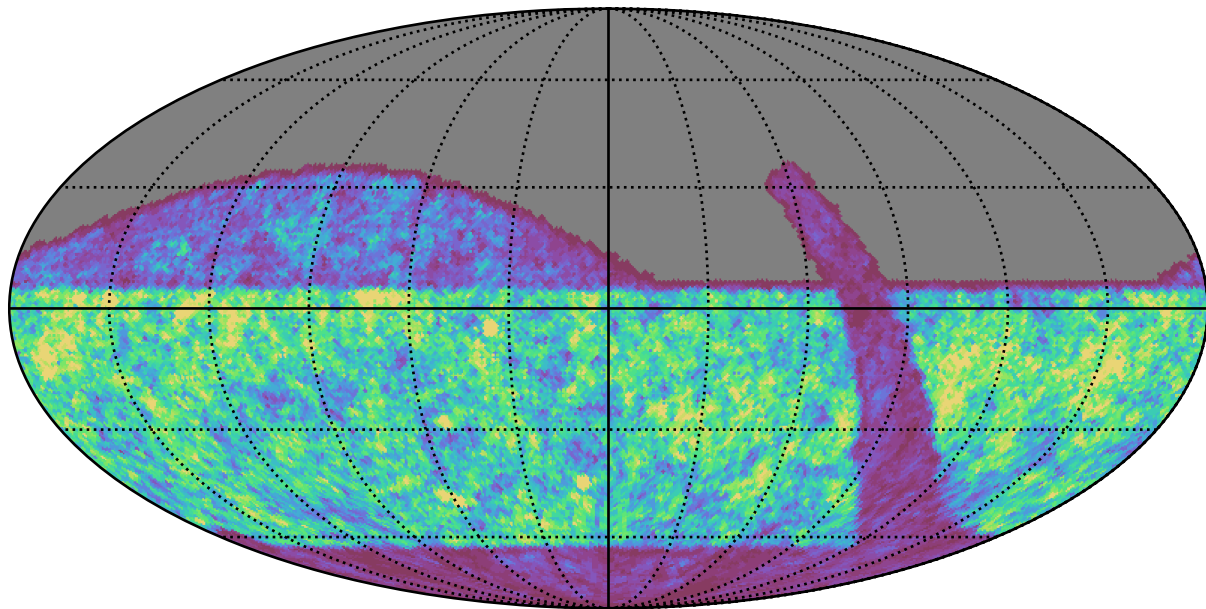
retro_baseline_v2.0_10yrs i band: Gaps_24hr
