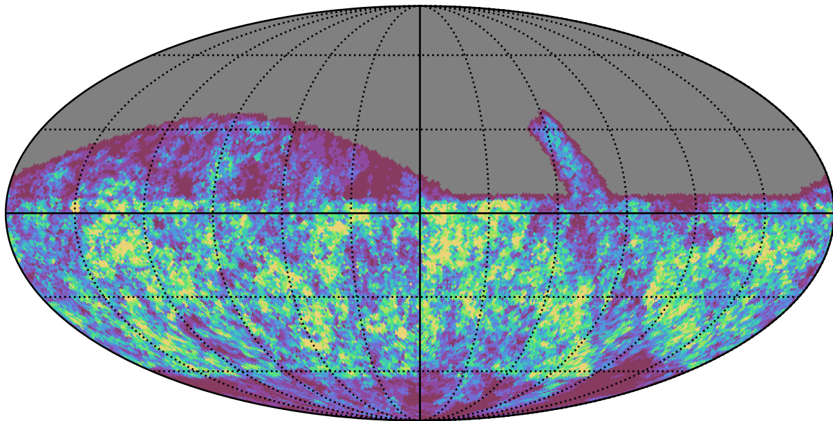
retro_baseline_v2.0_10yrs g band: Gaps_24hr
