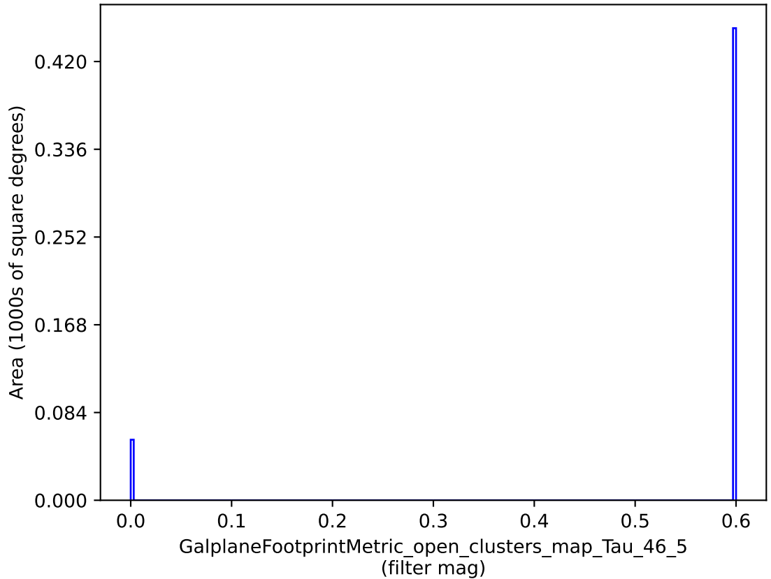
retro_baseline_v2.0_10yrs : GalplaneFootprintMetric_open_clusters_map_Tau_46_5
