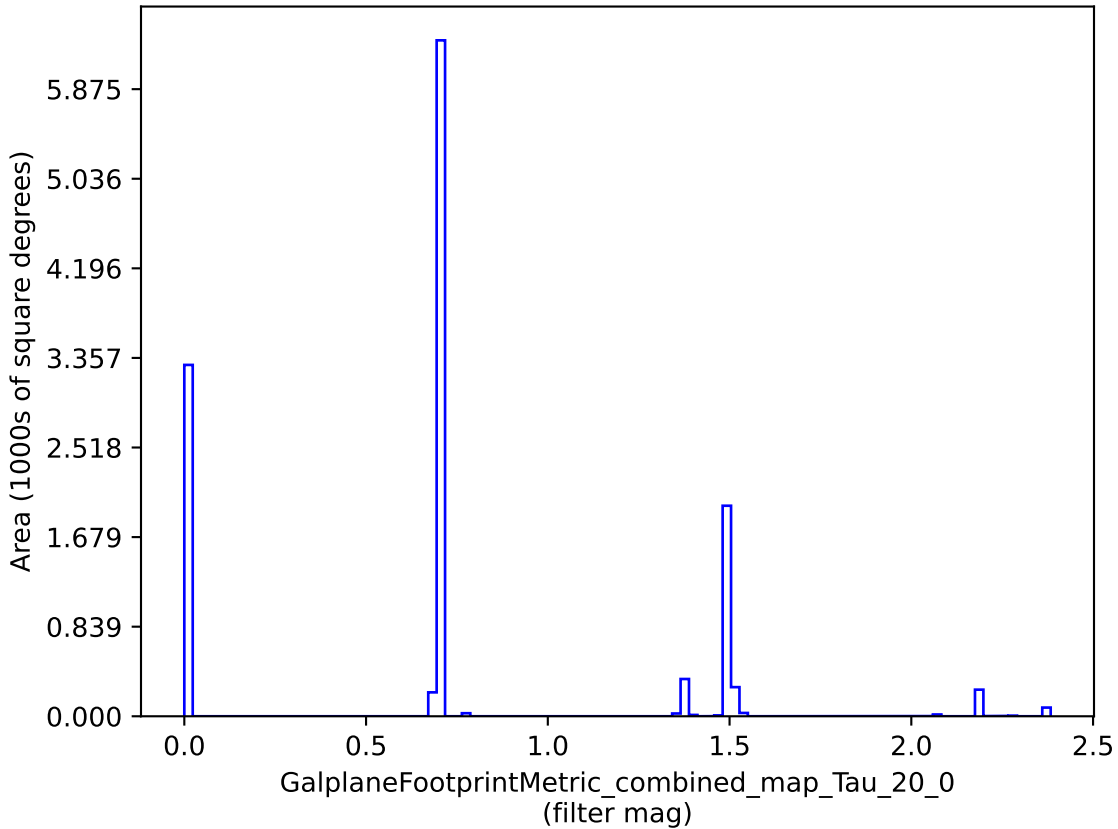
retro_baseline_v2.0_10yrs : GalplaneFootprintMetric_combined_map_Tau_20_0
