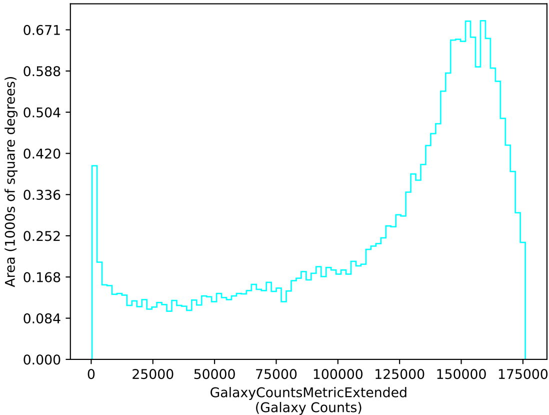
retro_baseline_v2.0_10yrs u: GalaxyCountsMetricExtended
