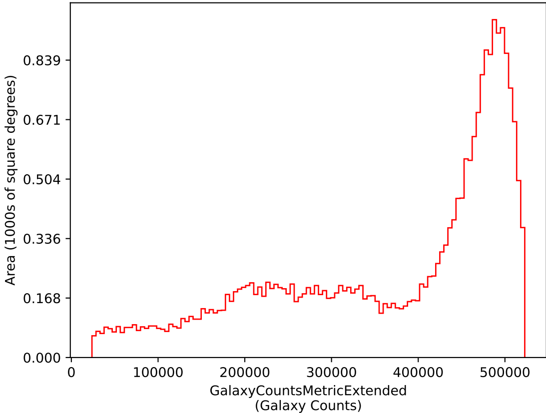
retro_baseline_v2.0_10yrs i: GalaxyCountsMetricExtended
