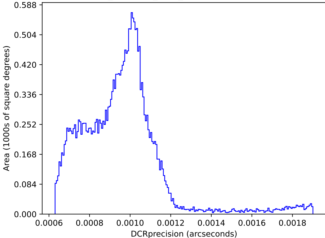
retro_baseline_v2.0_10yrs : DCRprecision
