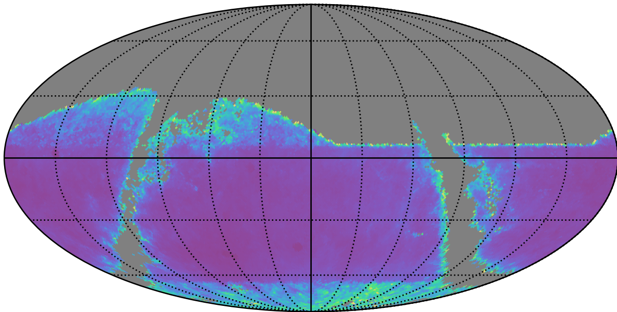
retro_baseline_v2.0_10yrs z band: AGN SF_uncert
