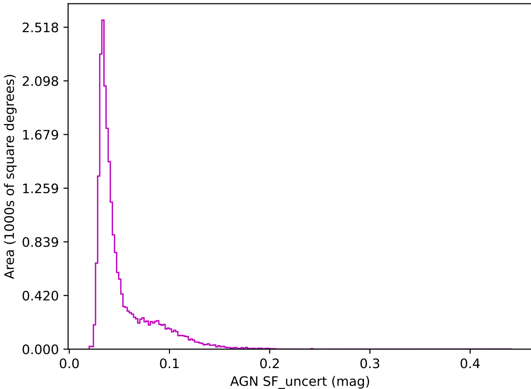
retro_baseline_v2.0_10yrs z band: AGN SF_uncert
