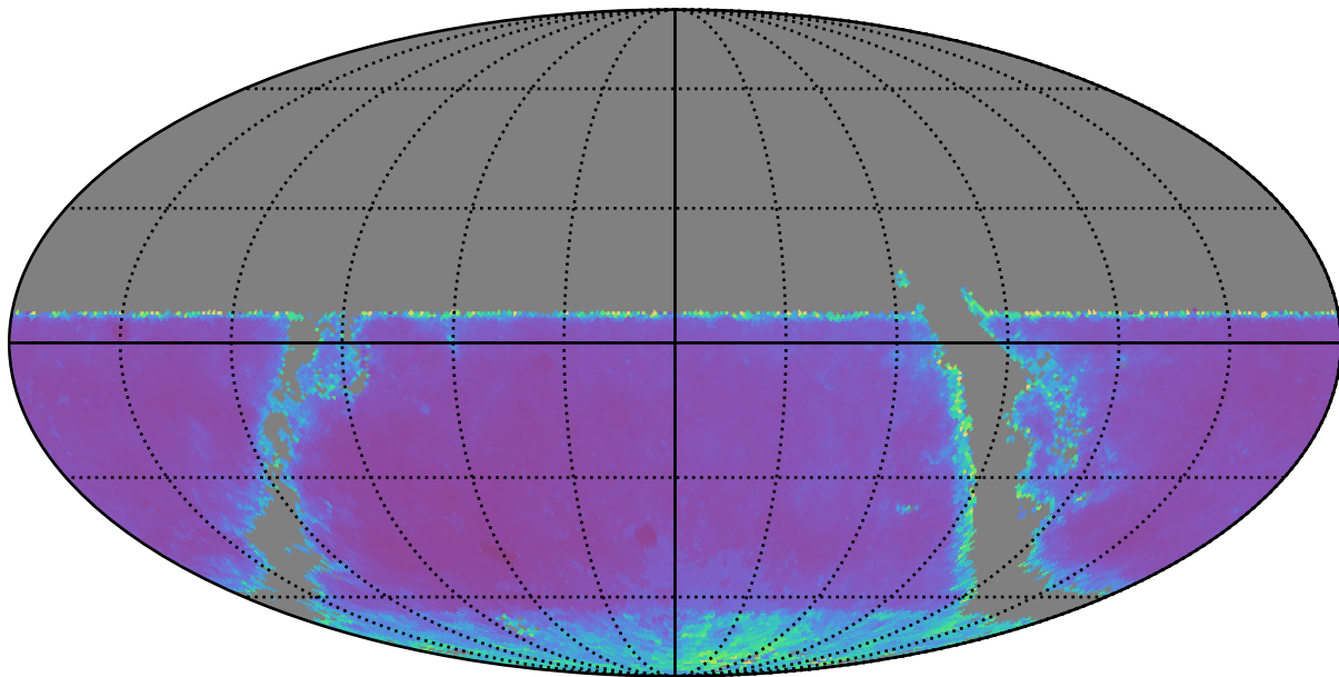
retro_baseline_v2.0_10yrs y band: AGN SF_uncert
