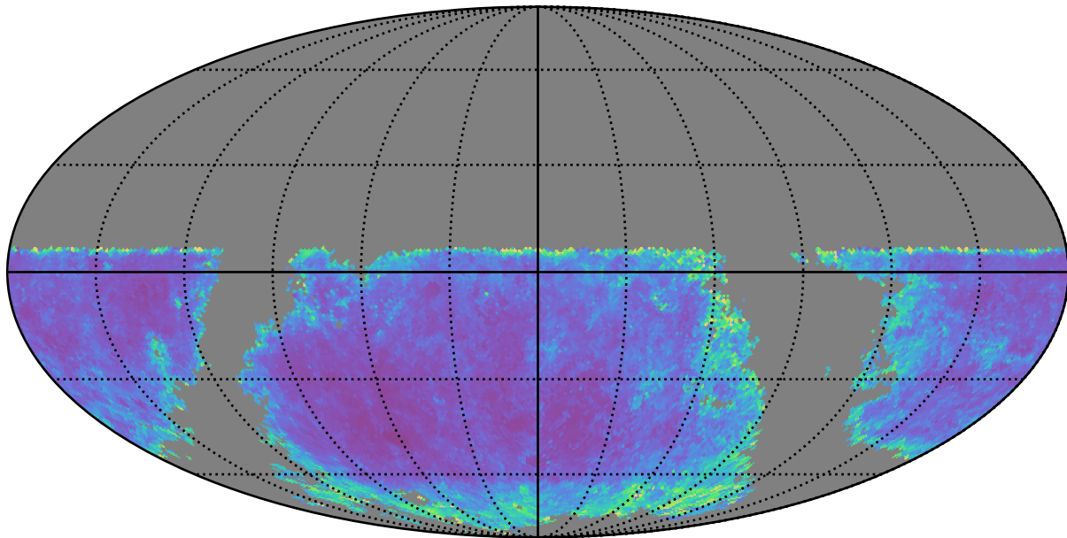
retro_baseline_v2.0_10yrs u band: AGN SF_uncert
