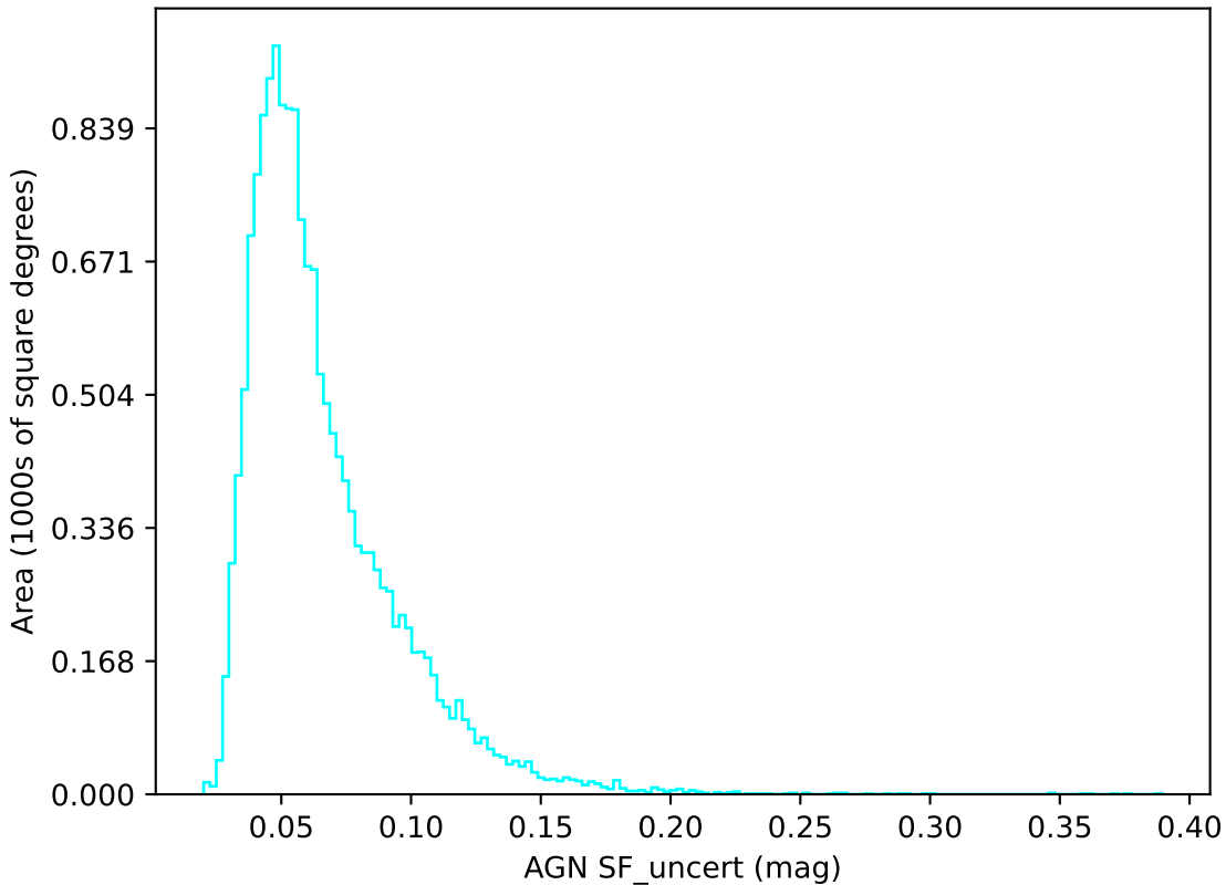
retro_baseline_v2.0_10yrs u band: AGN SF_uncert
