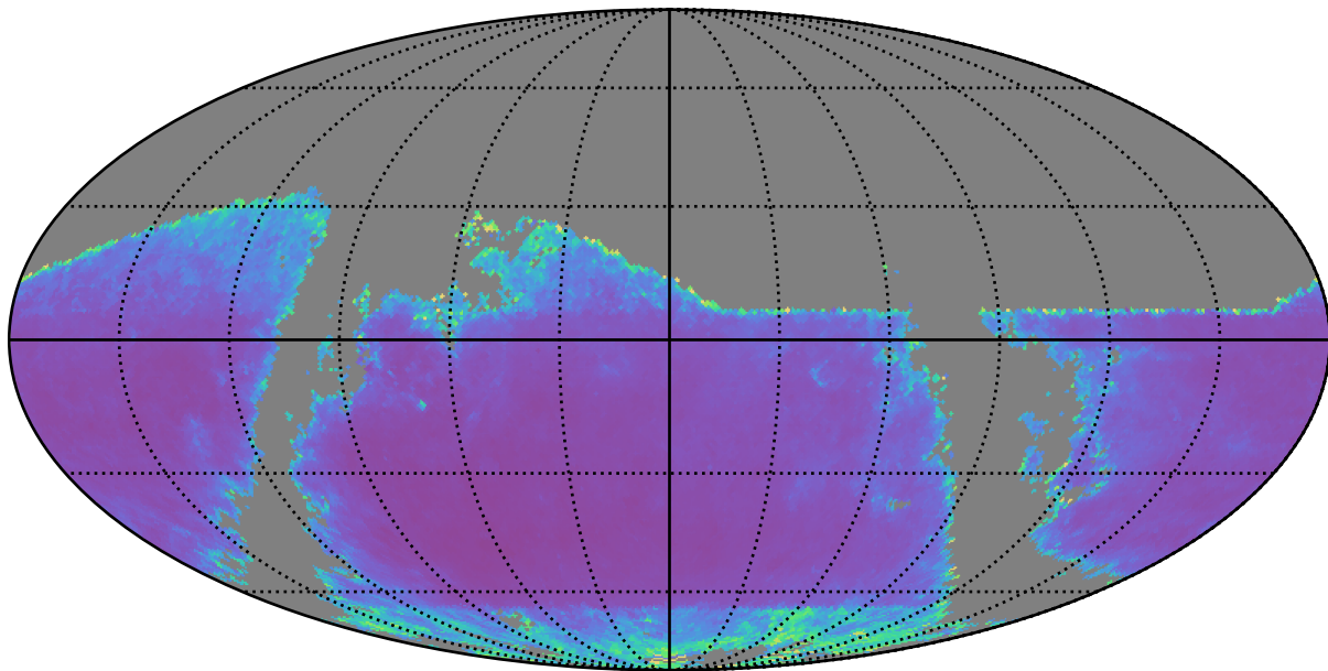
retro_baseline_v2.0_10yrs r band: AGN SF_uncert
