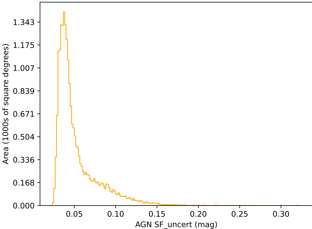
retro_baseline_v2.0_10yrs r band: AGN SF_uncert
