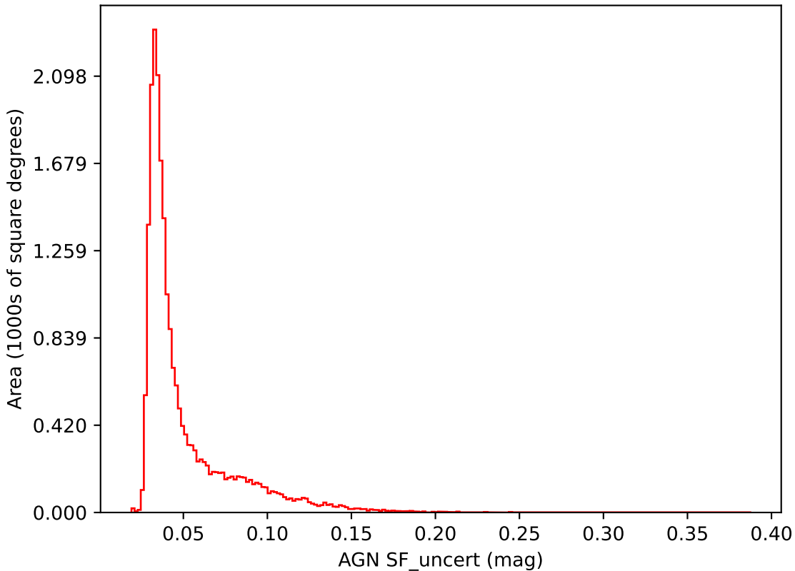
retro_baseline_v2.0_10yrs i band: AGN SF_uncert
