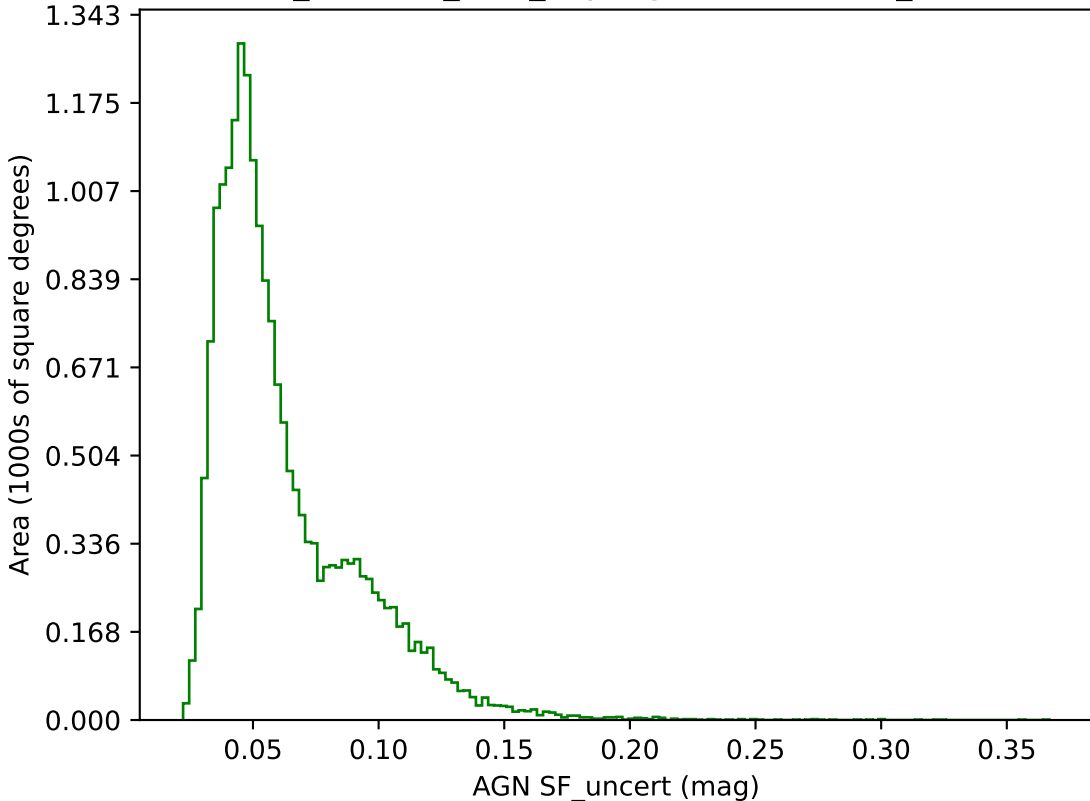
retro_baseline_v2.0_10yrs g band: AGN SF_uncert
