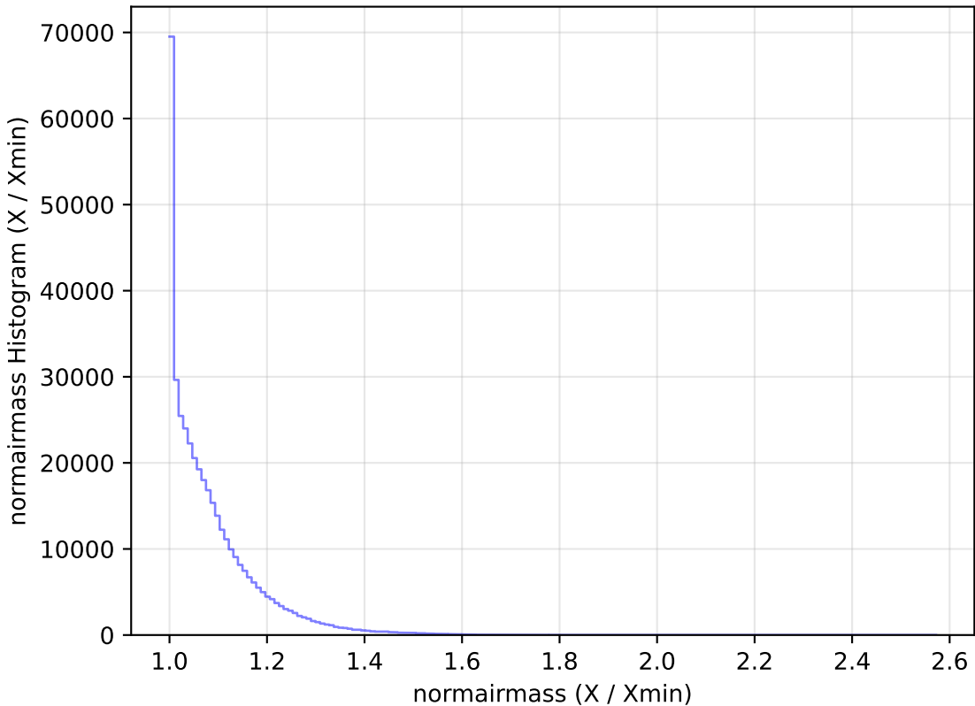
retro_baseline_v2.0_10yrs All sky y band: normairmass Histogram
