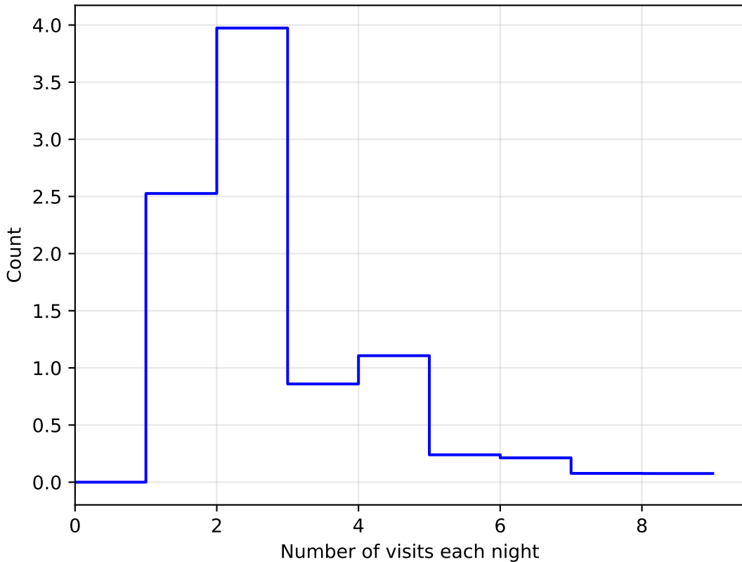
1e6 retro_baseline_v2.0_10yrs All sky: NVisitsPerNight
