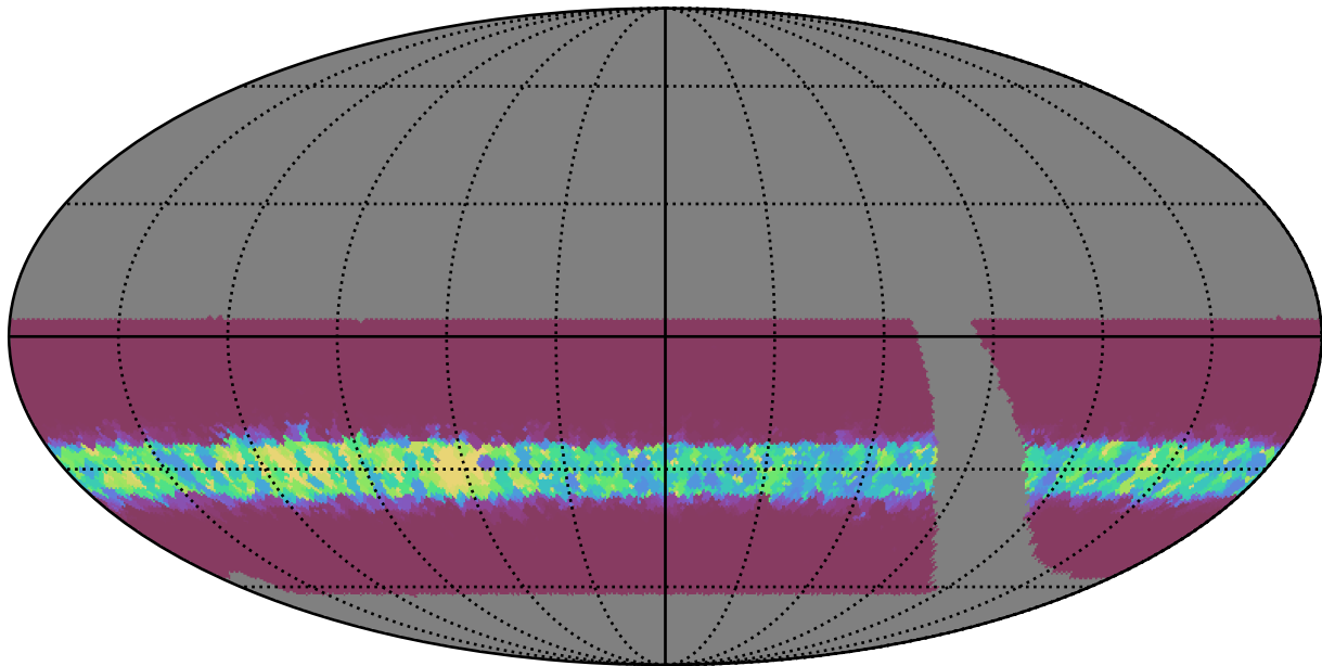
retro_baseline_v2.0_10yrs WFD z band: Min normairmass
