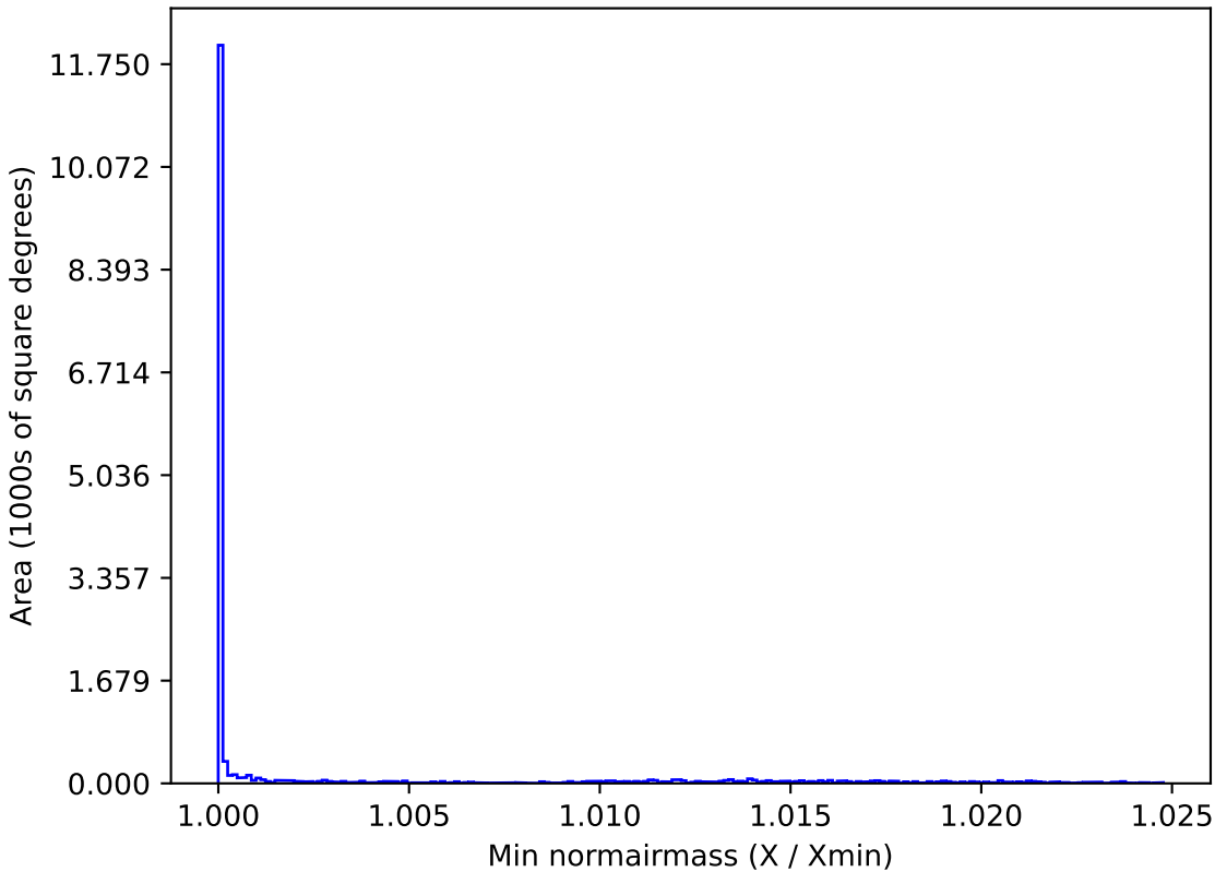
retro_baseline_v2.0_10yrs WFD z band: Min normairmass
