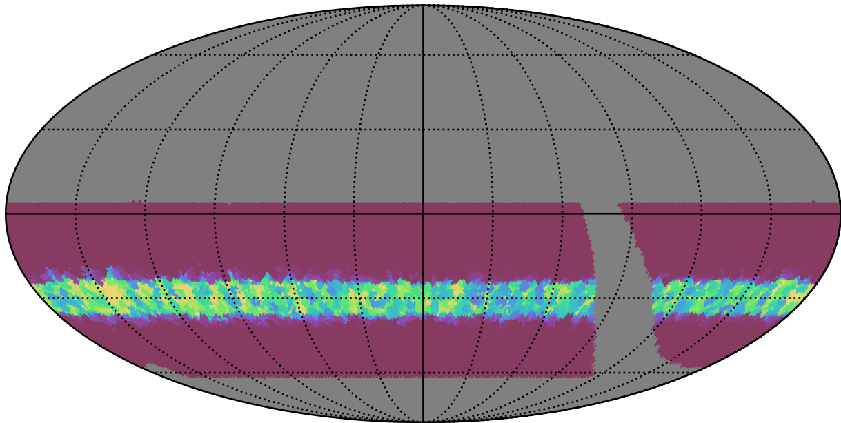
retro_baseline_v2.0_10yrs WFD y band: Min normairmass
