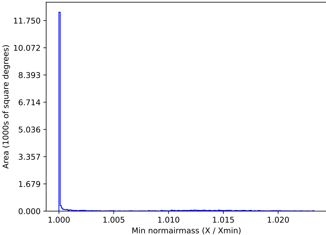
retro_baseline_v2.0_10yrs WFD r band: Min normairmass
