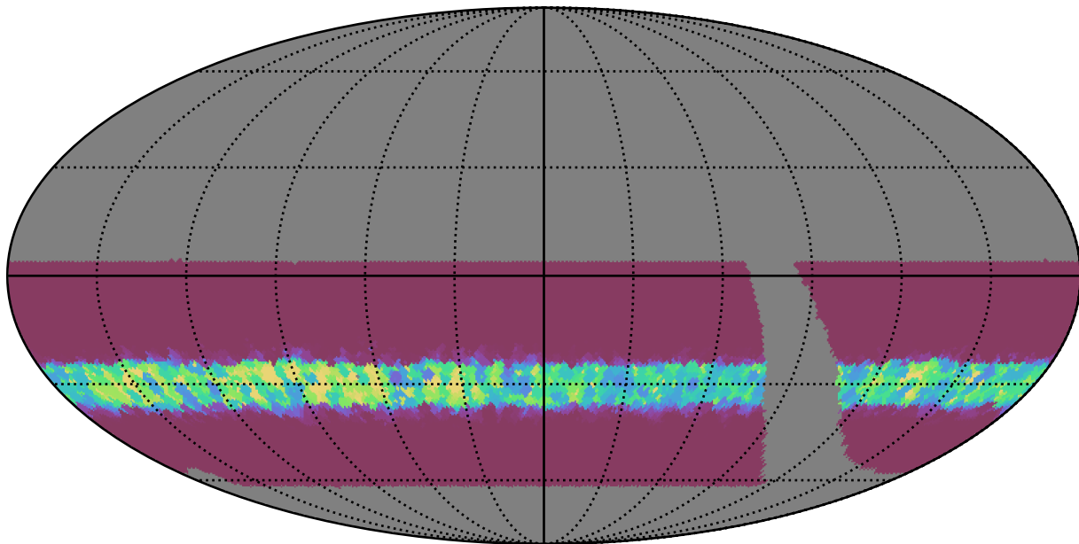
retro_baseline_v2.0_10yrs WFD i band: Min normairmass
