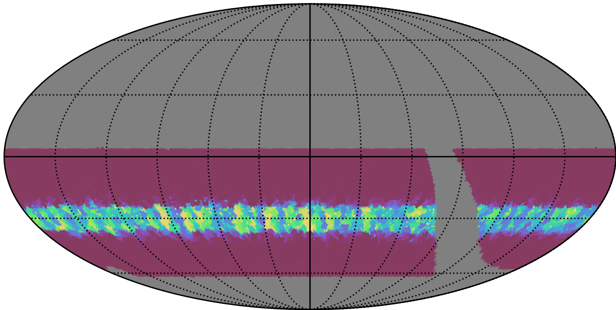
retro_baseline_v2.0_10yrs WFD g band: Min normairmass
