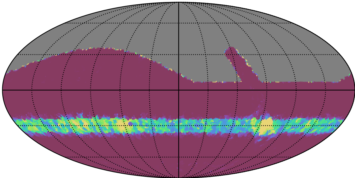
retro_baseline_v2.0_10yrs All sky z band: Min normairmass
