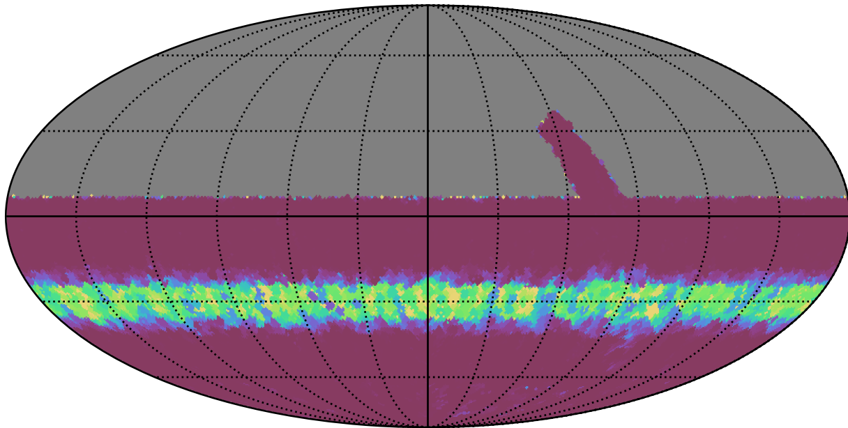
retro_baseline_v2.0_10yrs All sky u band: Min normairmass
