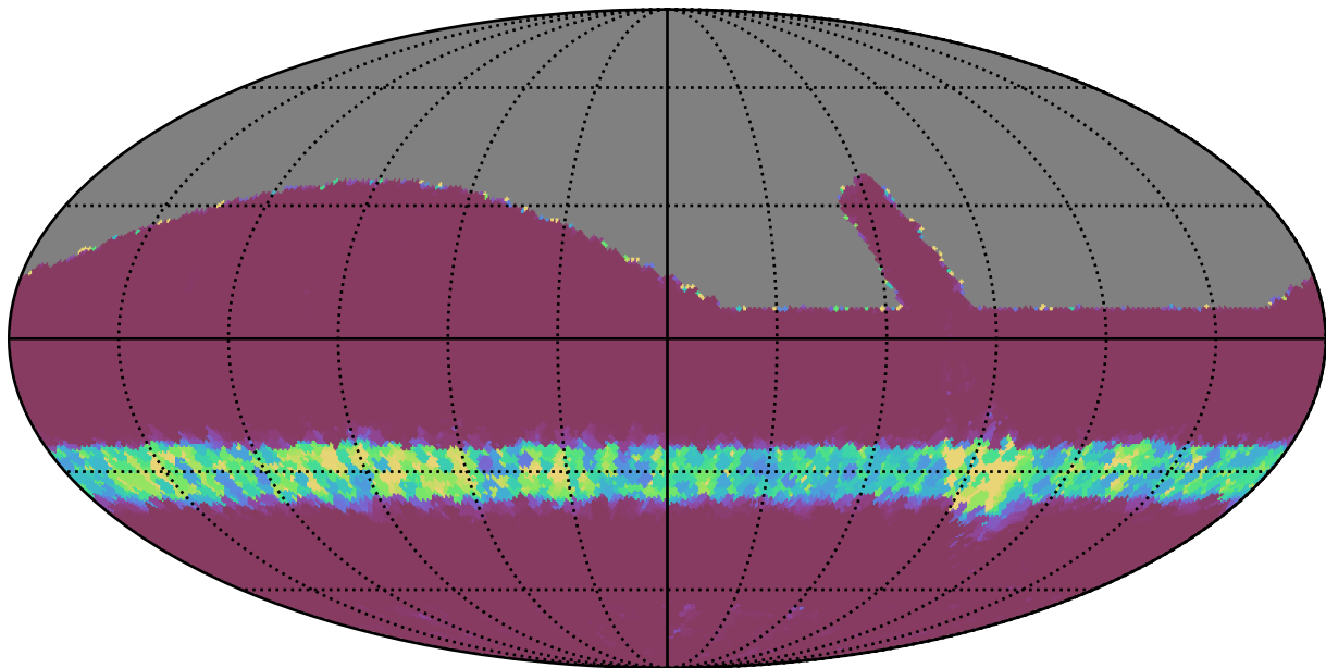
retro_baseline_v2.0_10yrs All sky i band: Min normairmass
