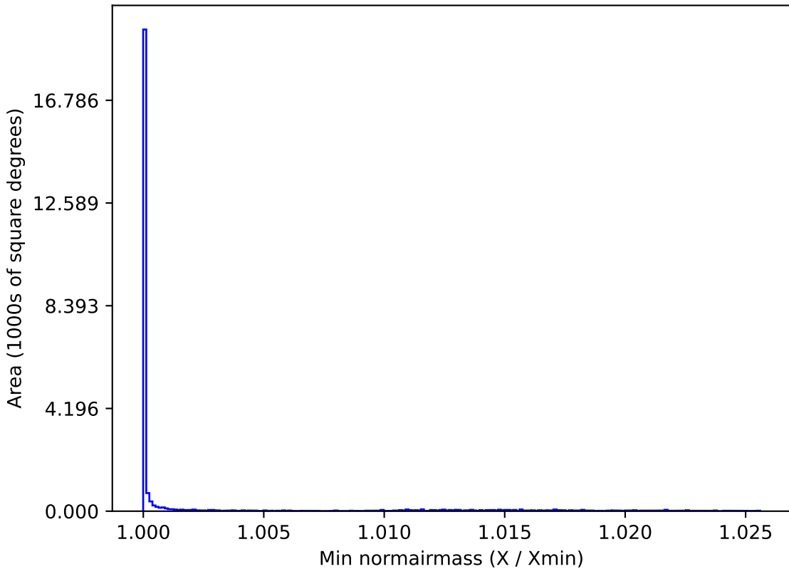
retro_baseline_v2.0_10yrs All sky i band: Min normairmass
