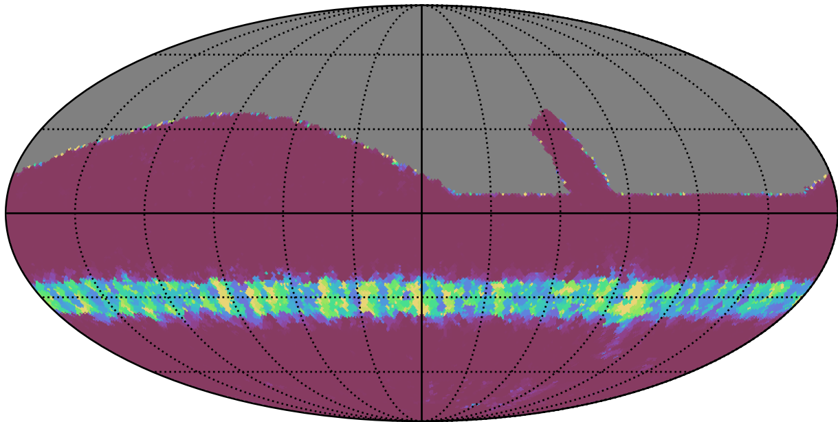
retro_baseline_v2.0_10yrs All sky g band: Min normairmass
