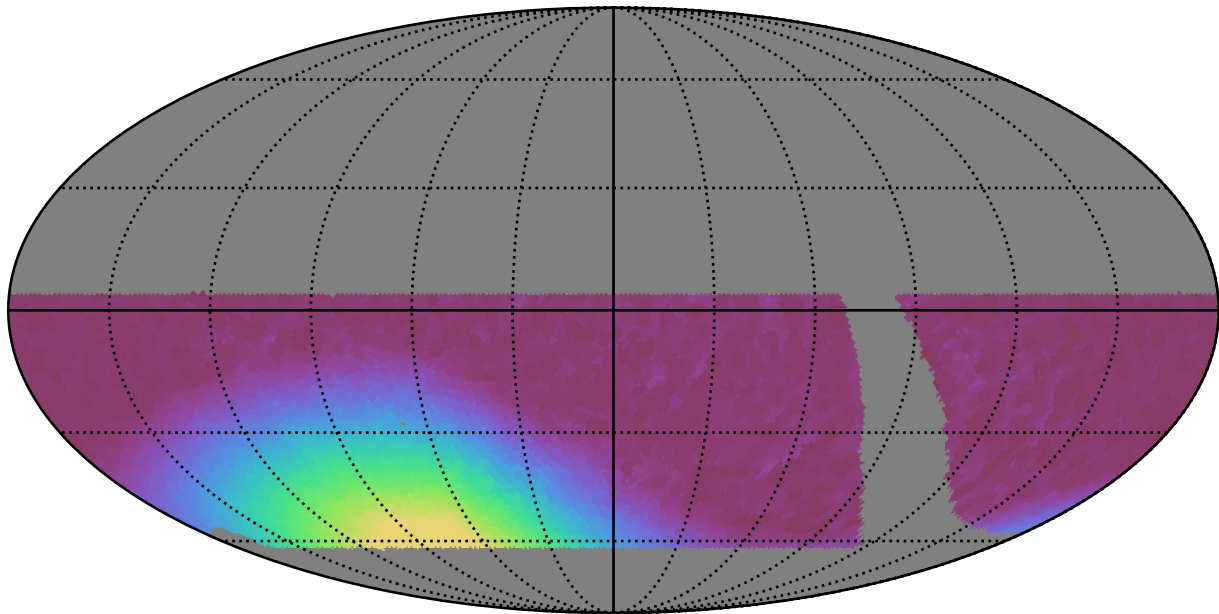
retro_baseline_v2.0_10yrs WFD y band: Min moonDistance
