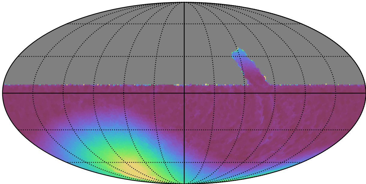
retro_baseline_v2.0_10yrs All sky y band: Min moonDistance
