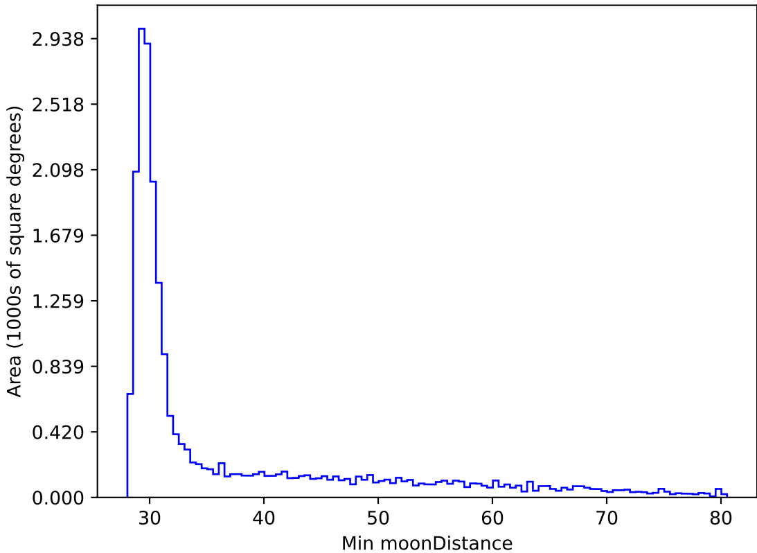
retro_baseline_v2.0_10yrs All sky y band: Min moonDistance
