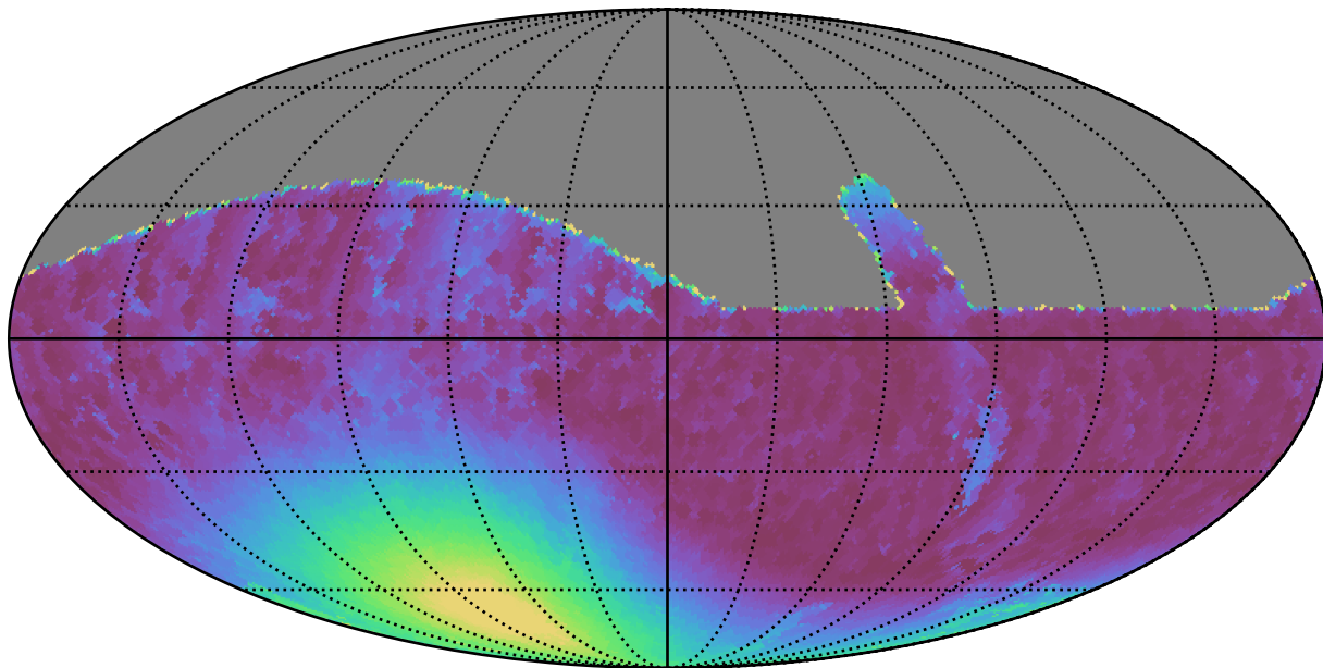
retro_baseline_v2.0_10yrs All sky i band: Min moonDistance
