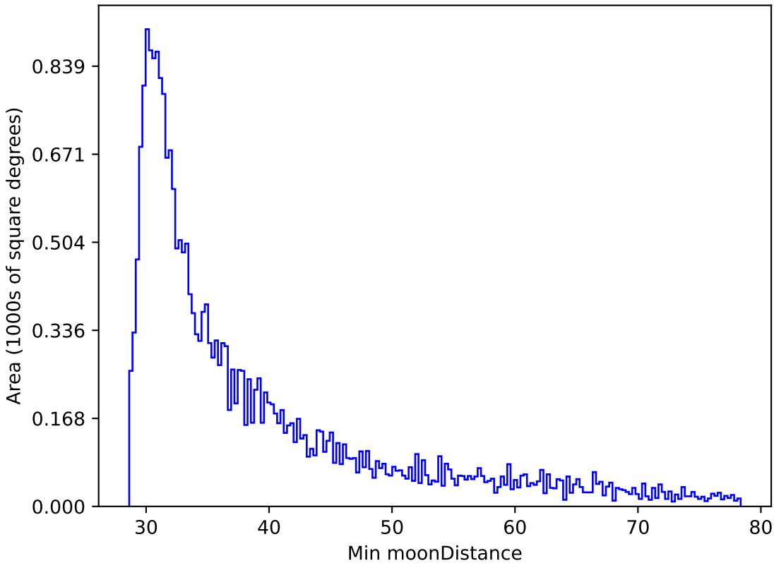
retro_baseline_v2.0_10yrs All sky i band: Min moonDistance
