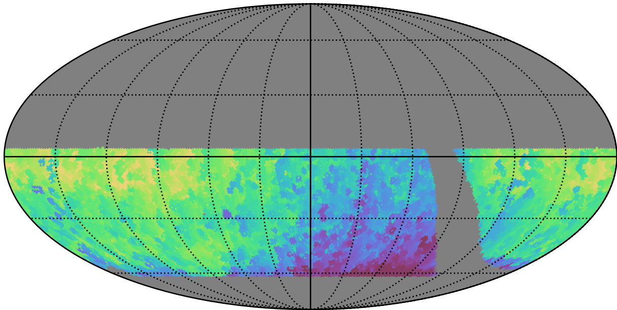
retro_baseline_v2.0_10yrs WFD z band: Min HA
